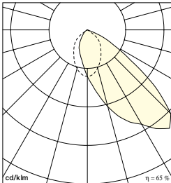
Fin Exterior 1 x 150W CDM-TD
