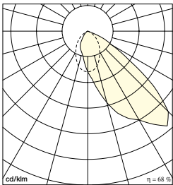
Fin Exterior 1 x 70W CDM-TD
